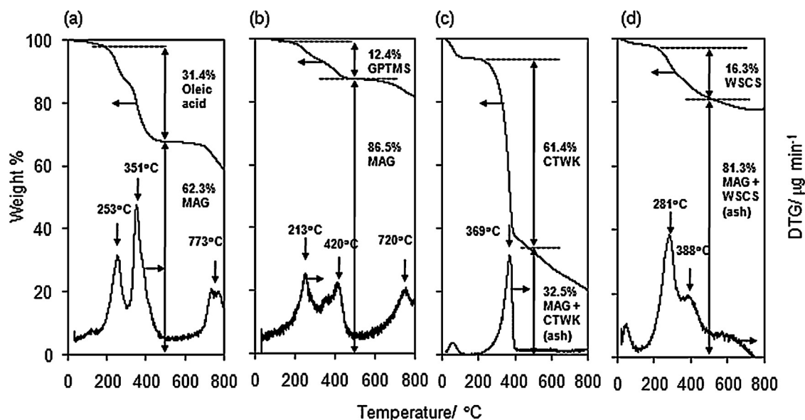
Fig. 2. TGA thermograms of (a) O-MAG, (b) S-MAG, (c) CTWK-MAG, and (d) WSCS-MAG.
